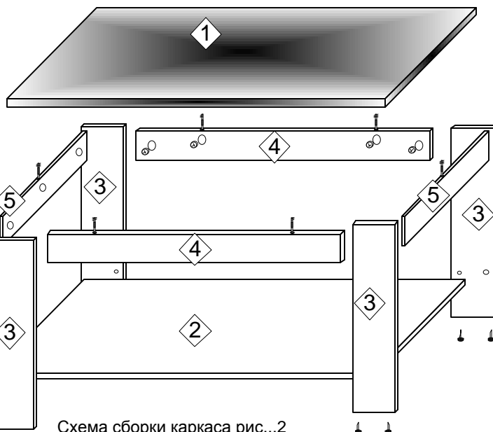
Схема сборки каркаса рис...2
