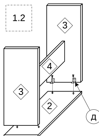
2 Схема установки опор и столешен
