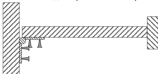
Схема установки петель на боковины для крепления опор
